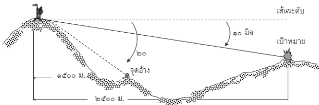
รูปที่ ๖ การคำนวณการย้ายทางดิ่ง (รูปไม่ถูกต้องตามมาตราส่วน)
