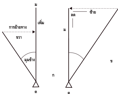
รูปที่ ๔ การกำหนดที่ตั้งเป้าหมายโดยวิธีย้ายจากจุดที่ทราบ
